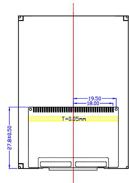
弯折参考图
